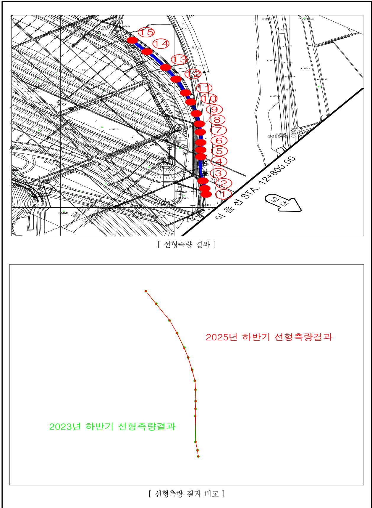
【그림 3.4.3】 선형측량 결과 및 비교
